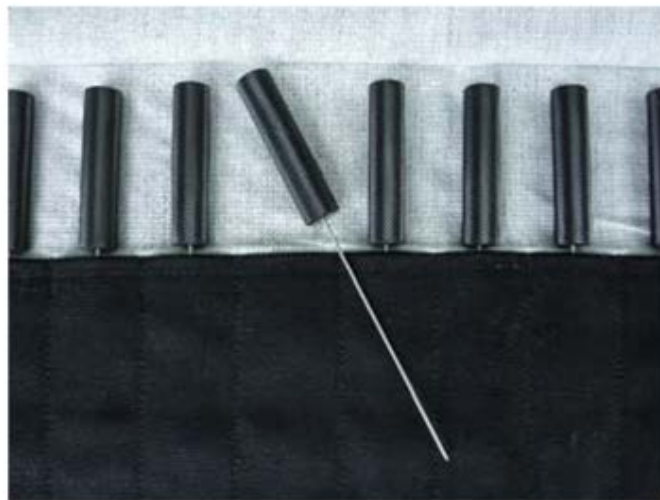
ソリッドブッシングバニッシャー (7種類)
